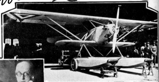
El general Juan F. AZCARATE, del Ejército mejicano, ha inventado este tren de aterrizaje, para aparatos anfíbios, que ha sido adoptado oficialmente por la Aviación Militar de Méjico, a causa de sus grandes ventajas. (Foto Underwood & Underwood).
